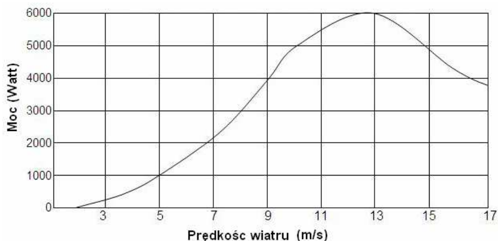
Rys. 3. Krzywa mocy dla turbiny 5kW
