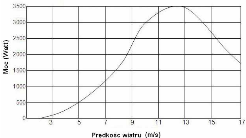
Rys.1. Krzywa mocy dla turbiny 3kW
